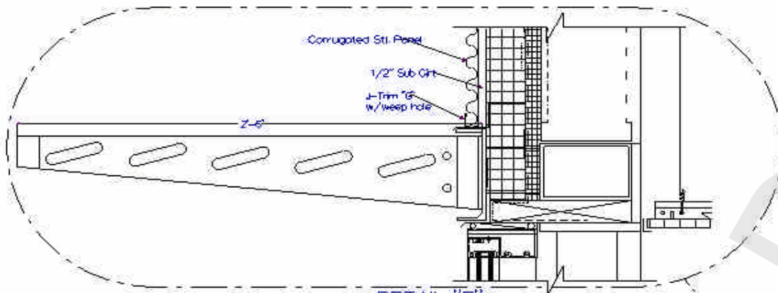
DETAIL "E" Scale: 3" = 1'-0"
